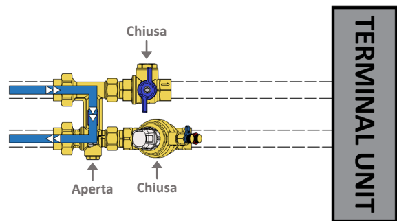
Modalità flushing: pulizia del circuito lato impianto
