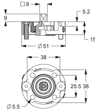
Vanne avec le moteur SN08 et l'accessoire de pré réglage 081PR1 installé
