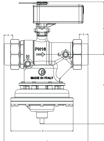
Vanne avec le moteur VA9208 - VA9208C et l'accessoire de pré réglage 081PR1 installé
