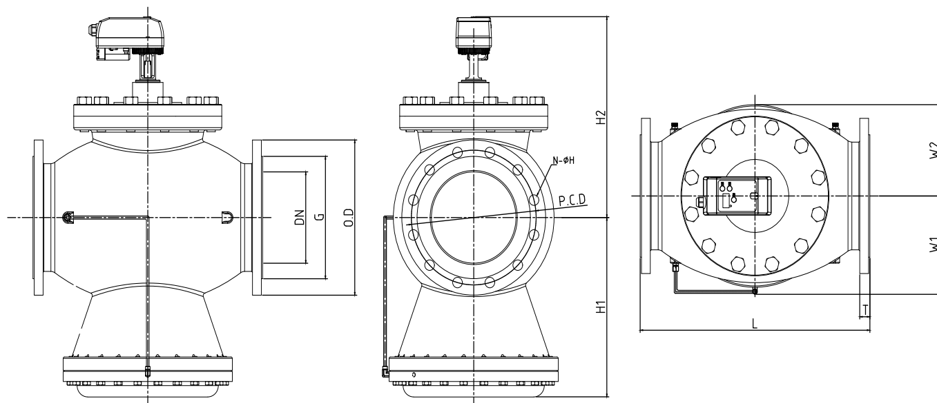
Vanne avec le moteur 24V
