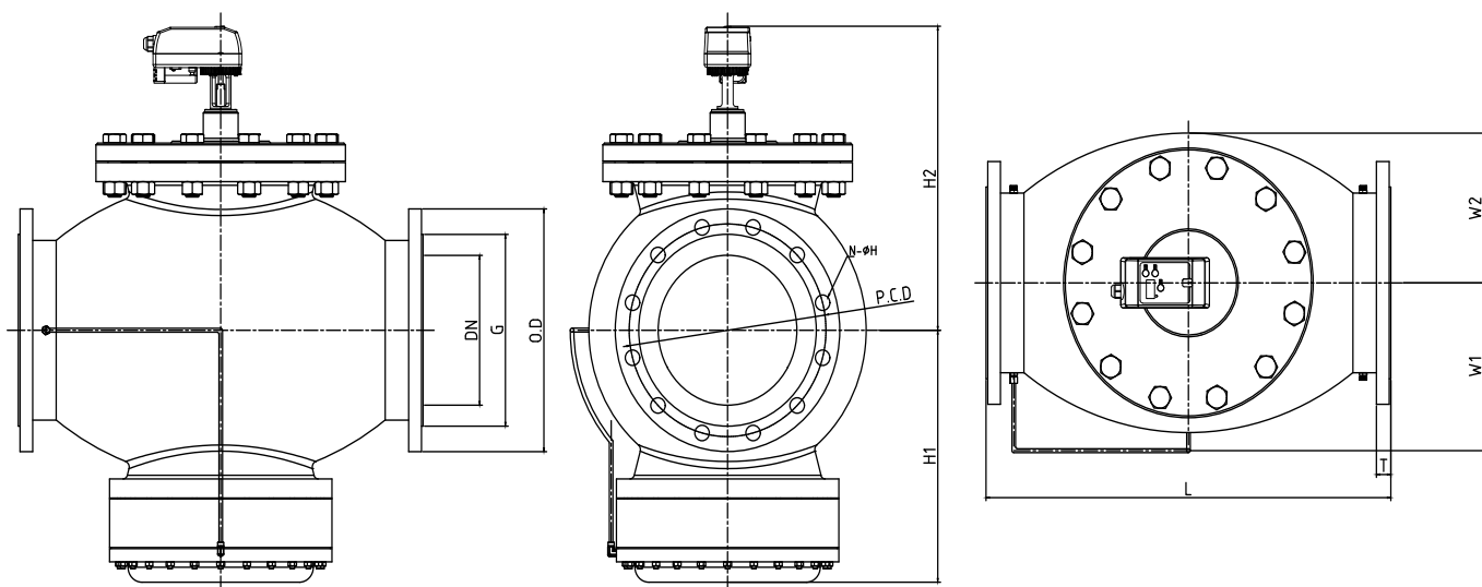
Vanne avec le moteur 24V
